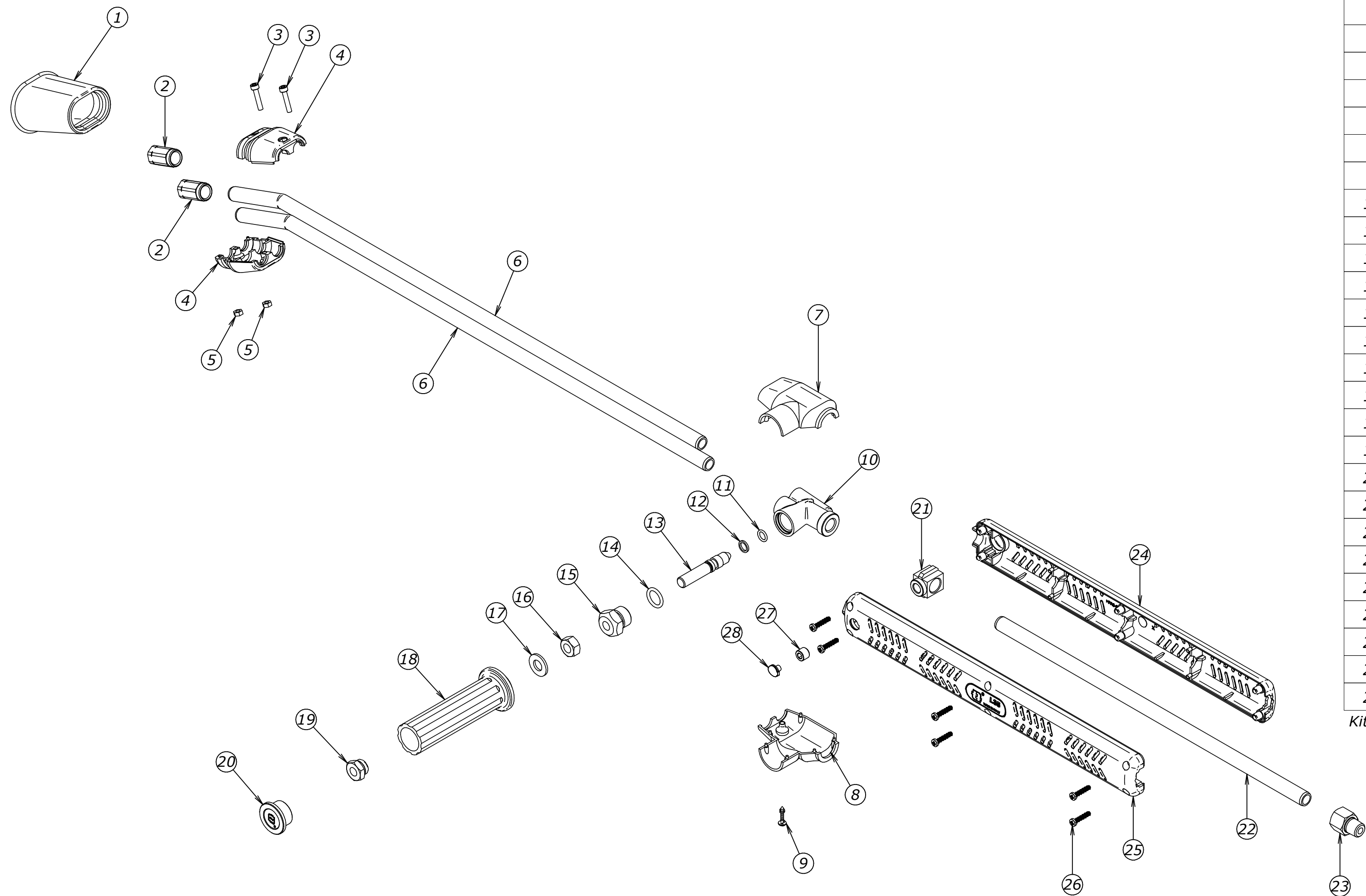
ESTREMITA' TUBO PIEGATO - BENT PIPE END
